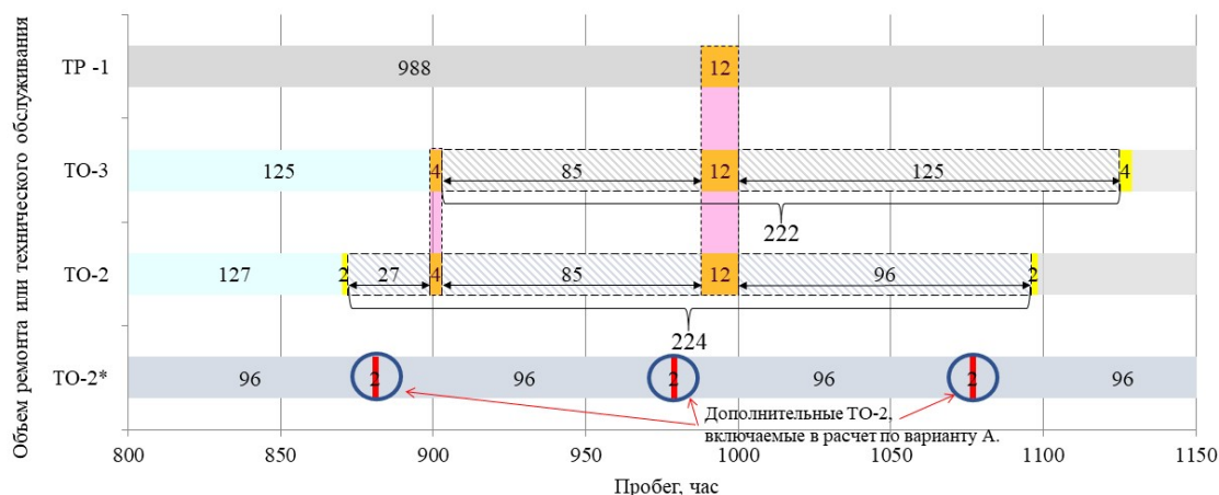
Рис. 5. Зависимость протяженности цикла ТО-2 от повторяемости циклов ТО-3
